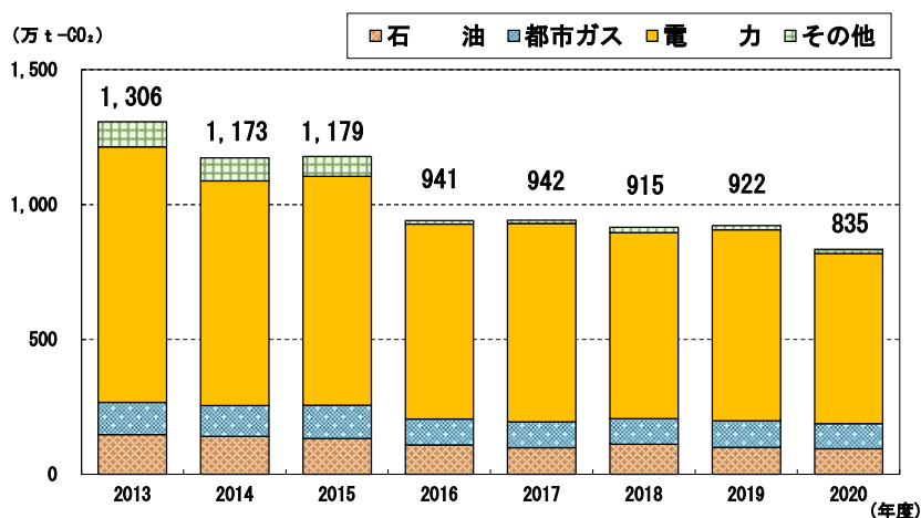
13 図2-3 CO 2 排出量の推移（業務部門）
