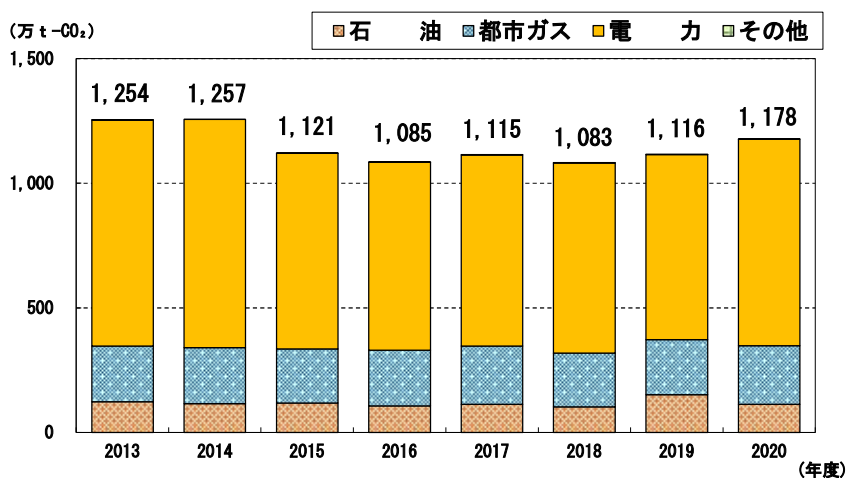
9 10 図2-4 CO 2 排出量の推移（家庭部門）
