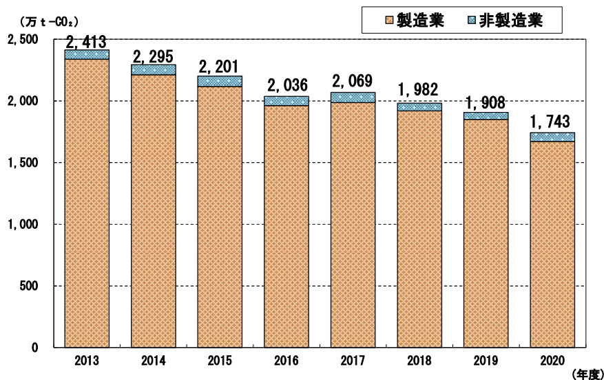
図2-2 CO 2 排出量の推移（産業部門）
