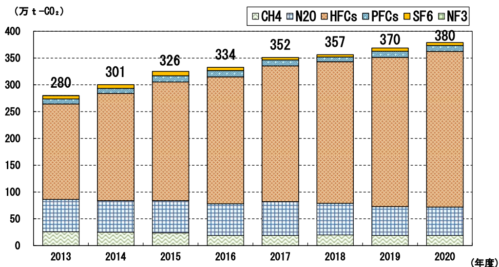
11 図2-7 その他ガス排出量の推移
