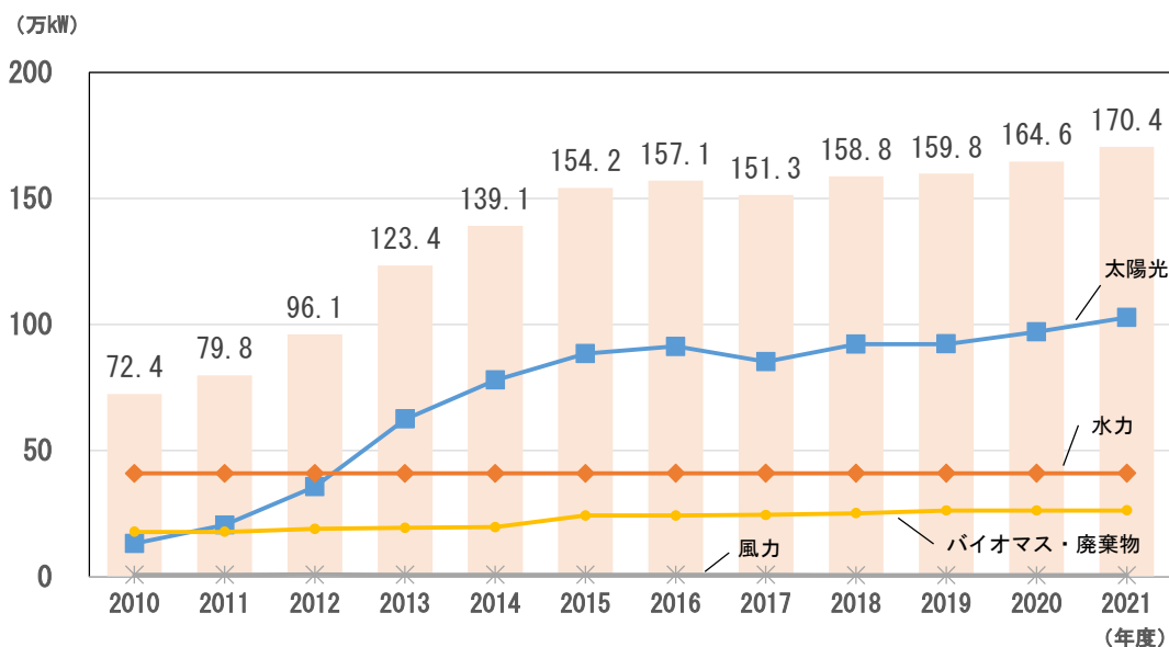
13 図1-8 県内の再生可能エネルギー別導入量の推移
