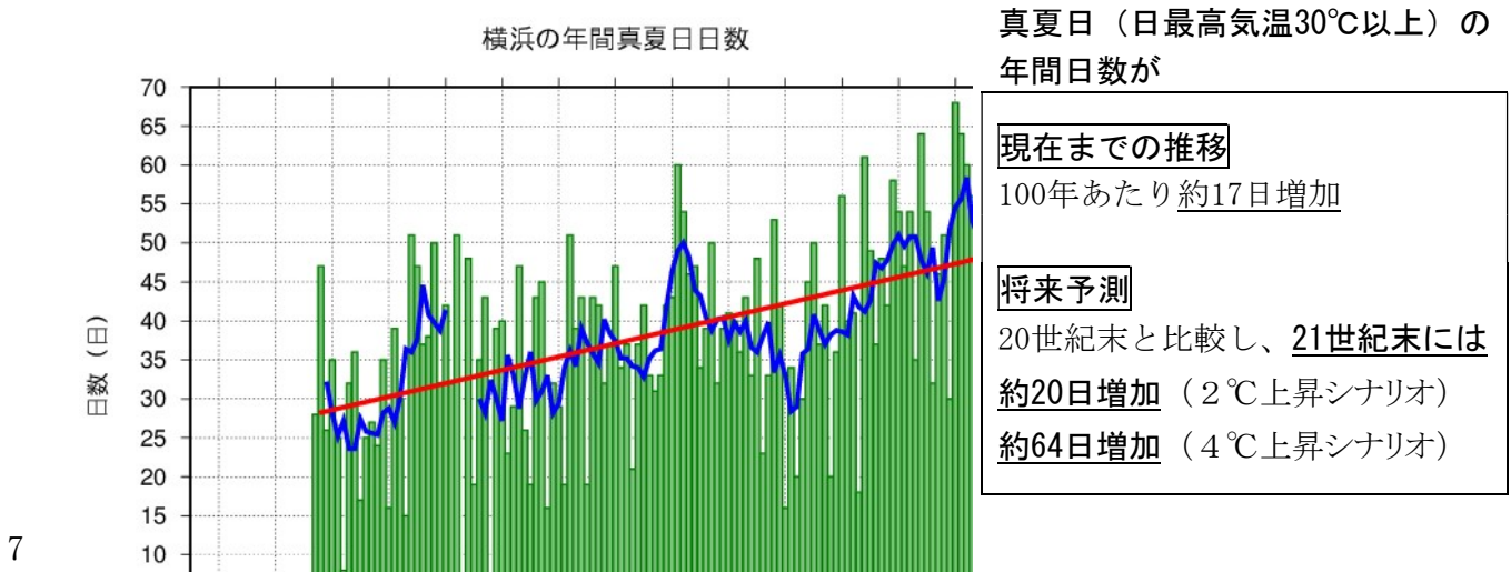
6 図3—2 横浜地方気象台における真夏日の日数の変化
