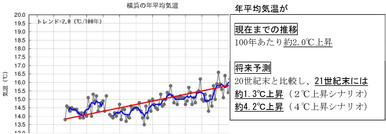
1 図3—1 横浜地方気象台における年平均気温の変化
