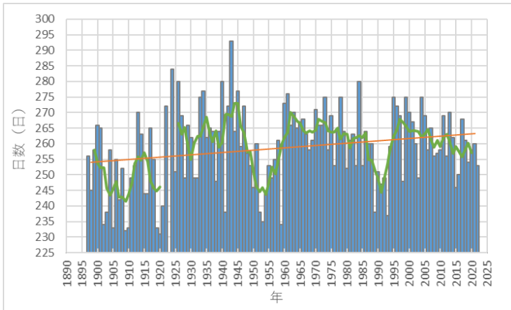
1 図3—4 横浜地方気象台における年間無降水の日数の変化
