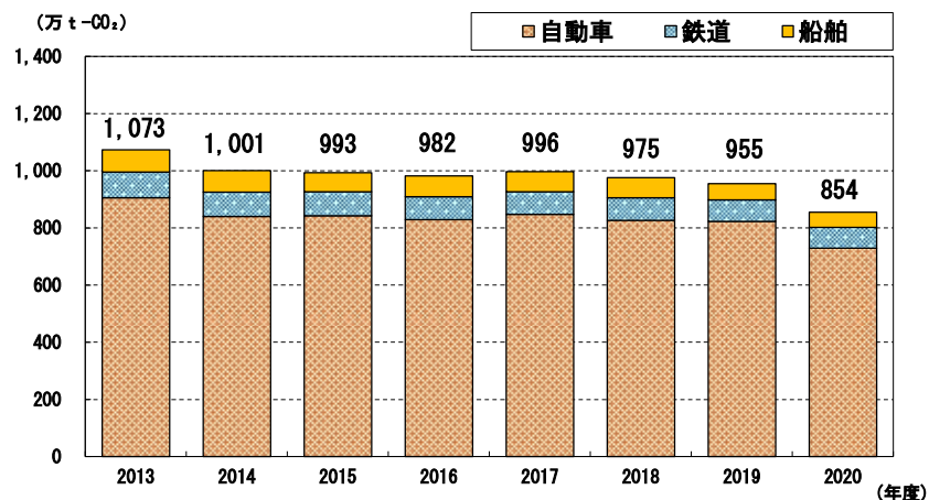
12 13 図2-5 CO 2 排出量の推移（運輸部門）
